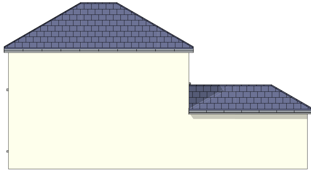
Pignon Gauche
