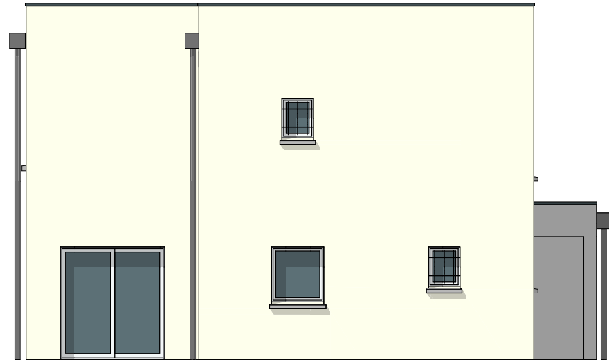
Pignon Gauche
